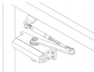
平行安装型 (P型) Parallel Arm Application
