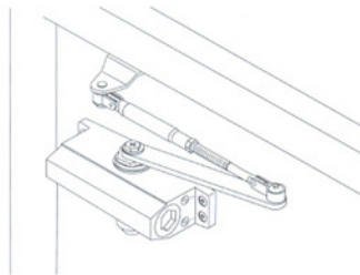
平行安装型 (P型) Parallel Arm Application
